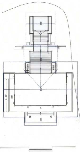
↑ 側面（社殿左側）からの間取り（案） 将来のバリアフリーを考えてスロープを付ける予定です。
