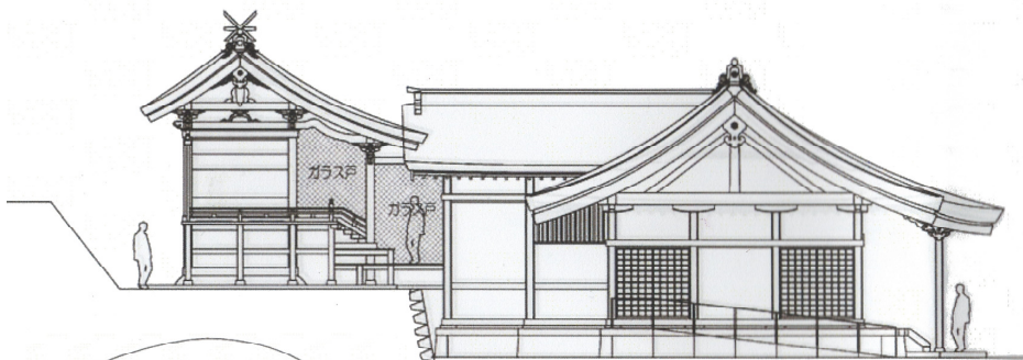
↑ 側面（社殿左側）からの間取り（案） 将来のバリアフリーを考えてスロープを付ける予定です。
