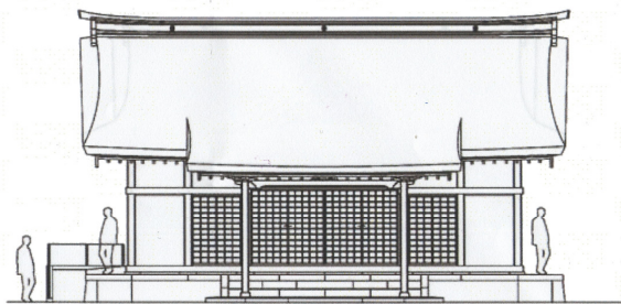
↑ 正面からの間取り（案） 現在は瓦の屋根ですが、銅板葺きに変更の予定です。
